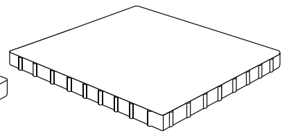
КВАДРАТ 1000 × 1000 1000 × 1000 × 100 мм
