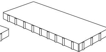
ПЛИТА 1000 × 500 × 80 мм 1000 × 500 × 100 мм
