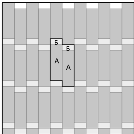
Паркет 600 x 200 - 85,7%(А), брусчатка 200 x 100 - 14,3%(Б)
