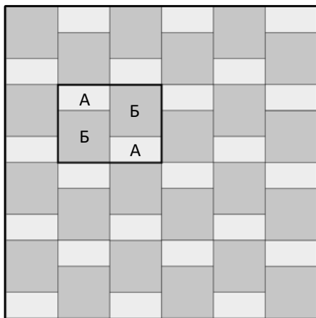
Брусчатка 200 x 100 - 33,3%(А), квадрат 200 x 200 - 66,7%(Б)
