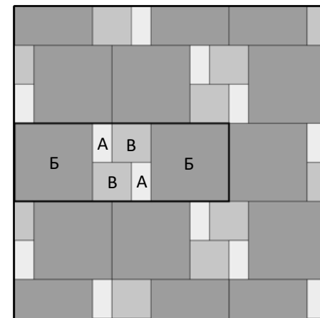
Брусчатка 200 x 100 - 9,1%, квадрат 400 x 400 - 72,72%, 200 x 200 - 18,18%
