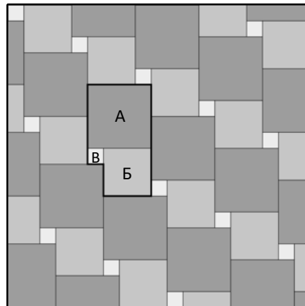
Квадрат 400 x 400 - 61,55%(А), 300 x 300 - 34,6%(Б), 100 x 100 - 3,85%(В)
