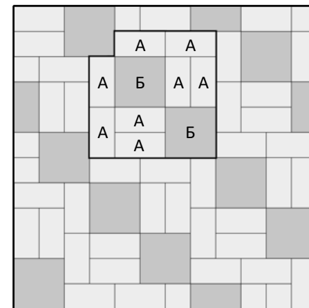
Брусчатка 200 x 100 - 60%(А), квадрат 200 x 200 - 40%(Б)
