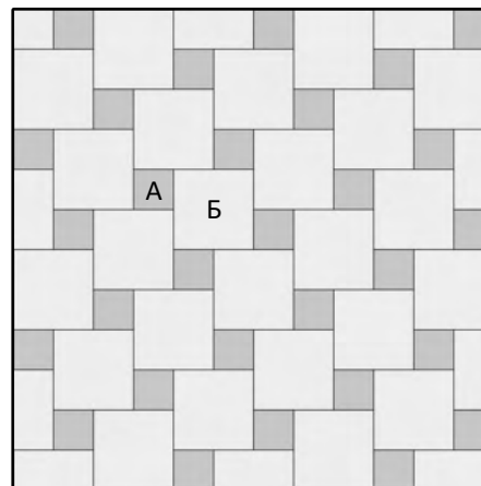
Квадрат 100 x 100 - 27%(А), 200 x 200 - 73%(Б)
