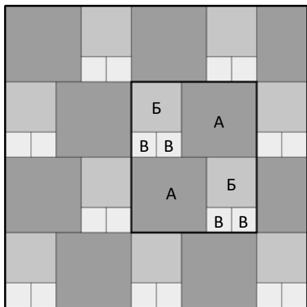
Квадрат 300 x 300 - 60%(А), 200 x 200 - 26,7%(Б), 100 x 100 - 13,3%(В)
