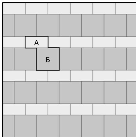
Брусчатка 200 x 100 - 66,7%(А), квадрат 200 x 200 - 33,3%(Б)
